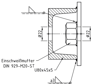
A-A M1:2
